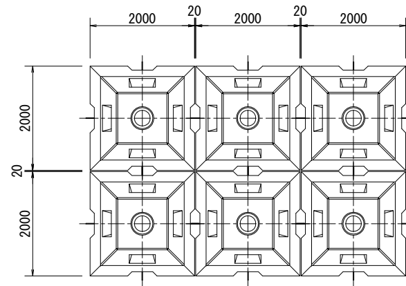
平面布設図
