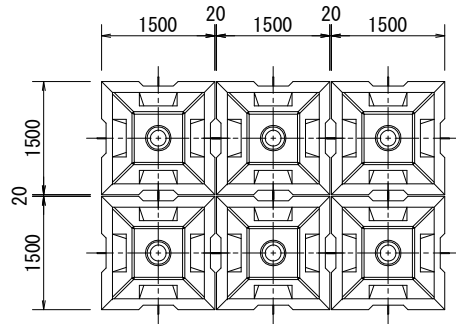
平面布設図
