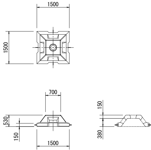
平面布設図
